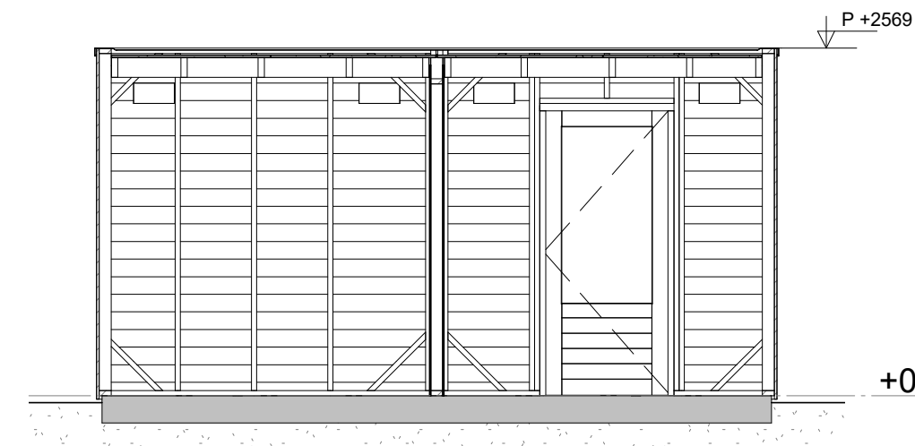
doorsnede B-B
